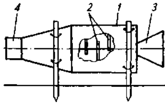
Рис. 6.4. Однокамерний пиловловлювач А.А. Знам'янського
