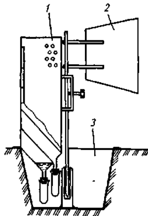
Рис. 6.5. Пилопісковловлювач УПЗ-50
