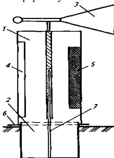
Рис 6.3. Пиловловлювач І.В. Годунова
